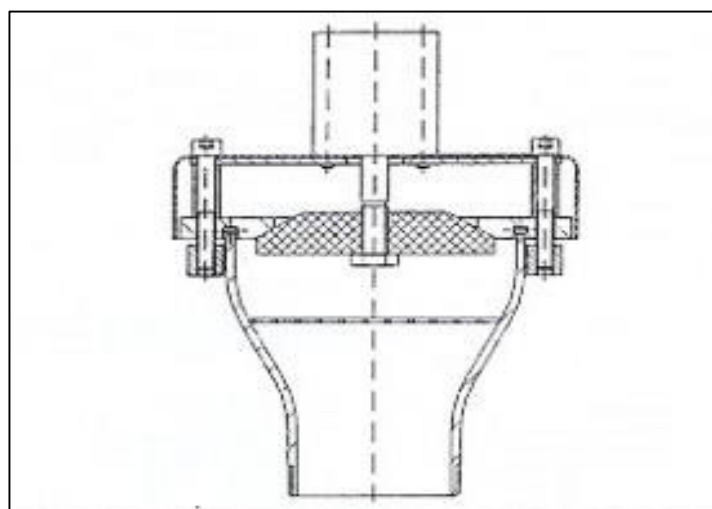
Slika 15. Shematski prikaz vakuumske crpke [5]
