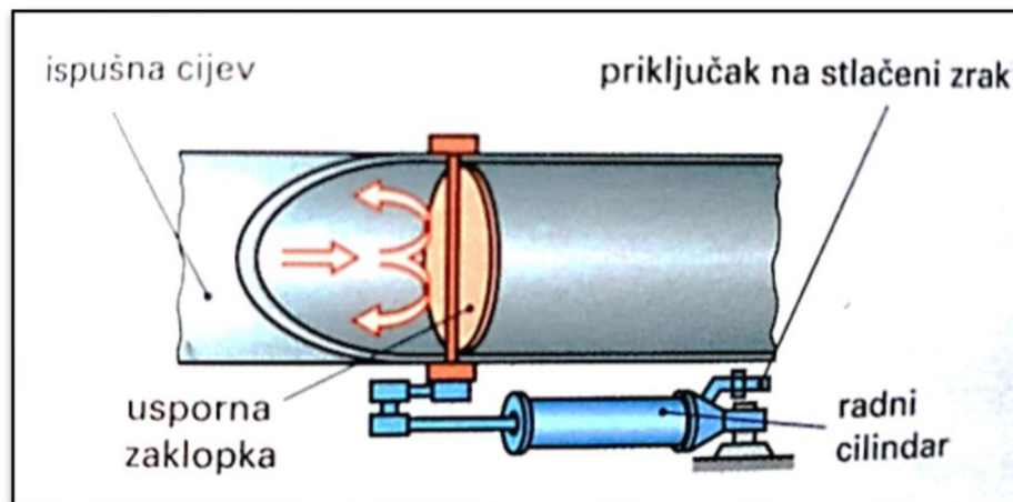
Slika 24. Shematski prikaz motorne kočnice.[2]
