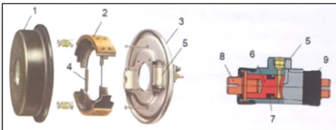
Slika 16. Shematski prikaz dijelova mehanizma bubanj kočnice. [1]
