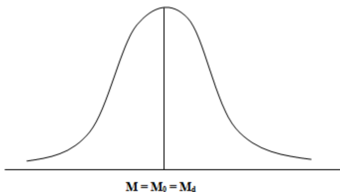
Slika 5. Simetrična unimodalna funkcija.
