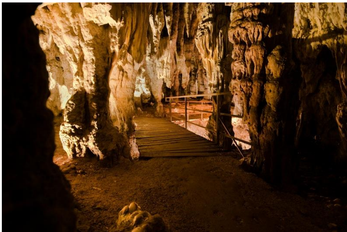
Slika 4. Baraćeve spilje
